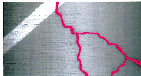
זיהוי אוטומטי של סדקים
